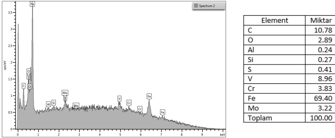
Şekil 3. Kriyojenik işlem görmüş numuneye ait EDS analizi
