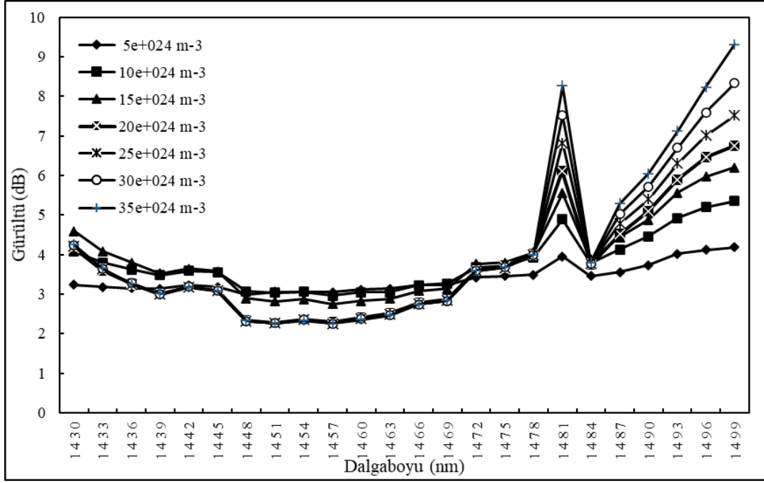
Şekil 7: Farklı iyon yoğunluklarında oluşan TKFY gürültü-dalgaboyu grafiği
