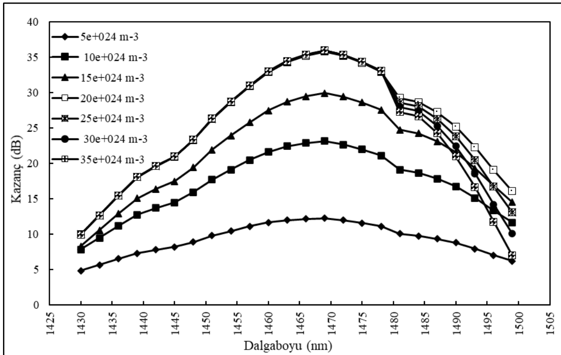
Şekil 6: Farklı iyon yoğunluklarında oluşan TKFY kazanç-dalgaboyu grafiği
