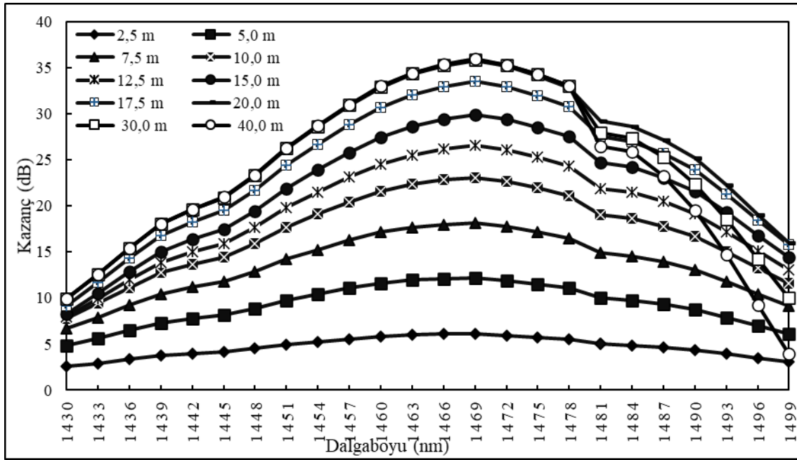
Şekil 4: Farklı TKF uzunluklarında oluşan TKFY kazanç-dalğaböyü
