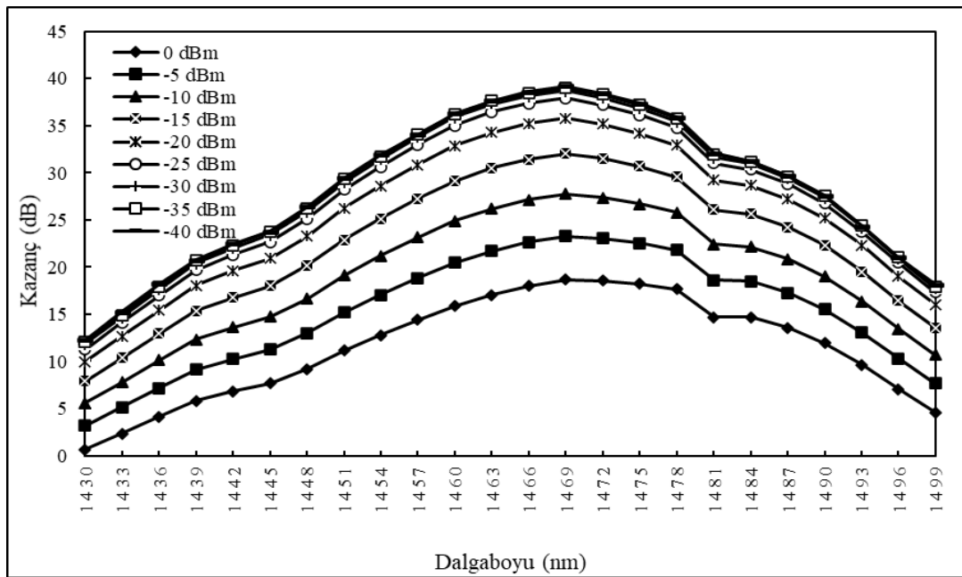
Şekil 8: Farklı giriş güçlerinde oluşan TKFY kazanç - dalgaboyu grafiği
