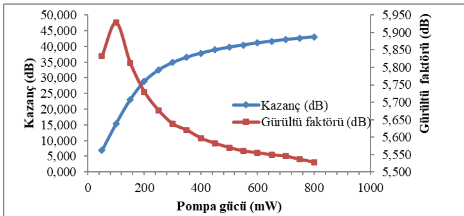
Şekil 3. Farklı pompa lazer güçleri için PKFA’nın çıkış kazancı ve gürültü etkisi
