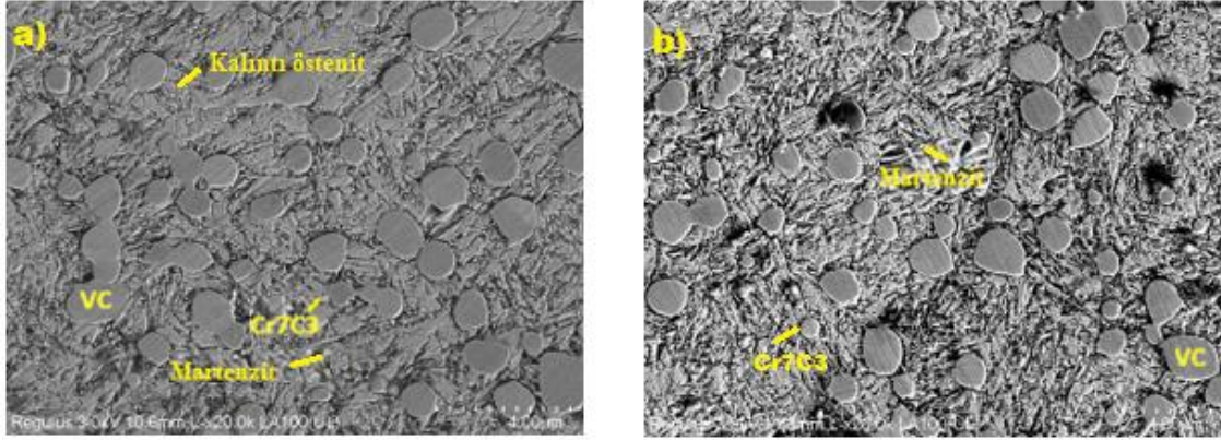
Şekil 1. Numunelere ait SEM mikroyapıları (x20.000)
