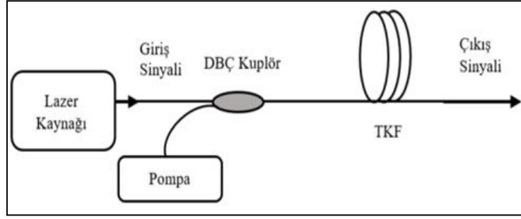
Şekil 1: Temel TKFY Tasarımı
