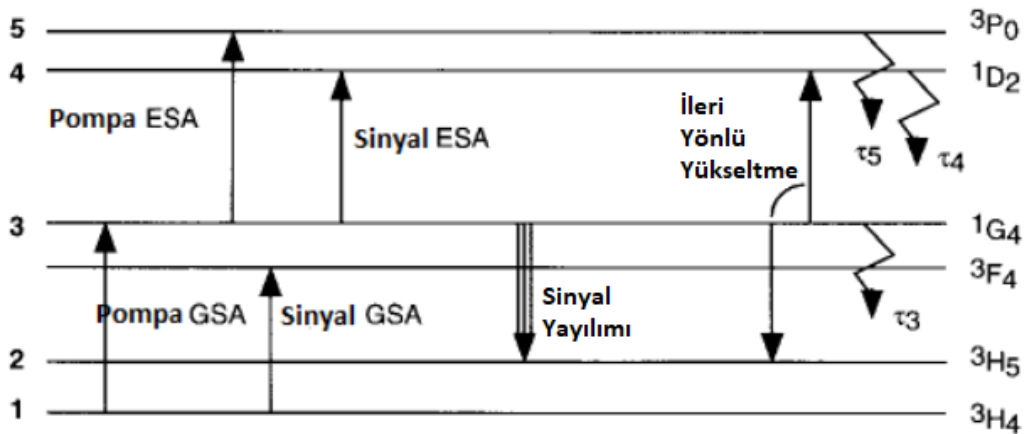
Şekil 1. Basitleştirilmiş praseodimyum enerji yapısı [12]
