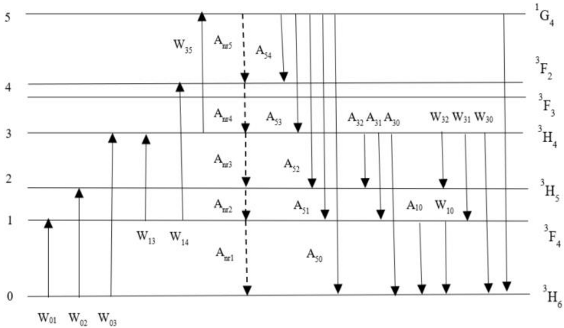
Şekil 2: Tulyum iyonlarının detaylı enerji diyagramı
