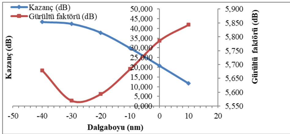
Şekil 4. Farklı giriş sinyal güçleri için PKFA'nın çıkış kazancı ve gürültü etkisi
