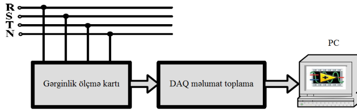
Şək. 1. İnformasiya-ölçmə sistemi
