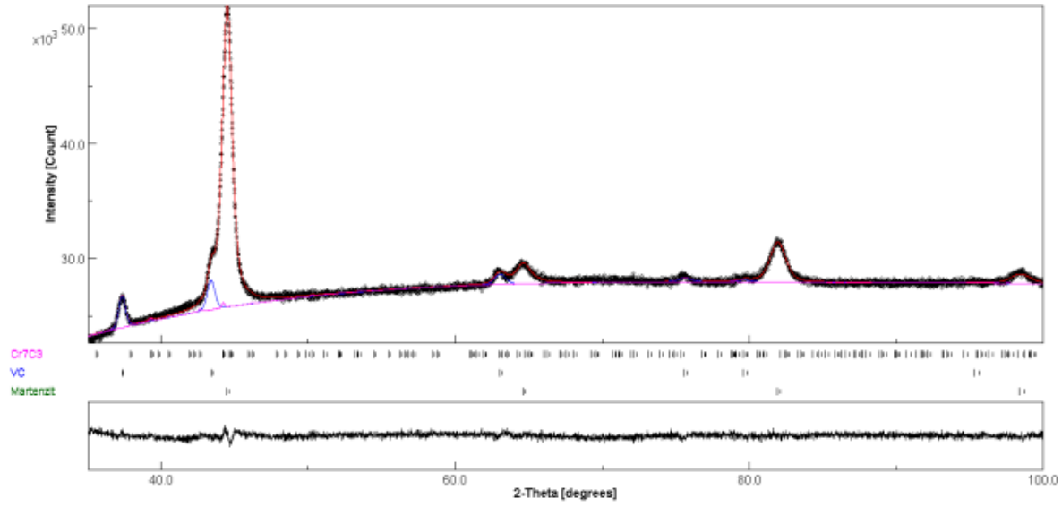
Şekil 5. Kriyojenik işlem görmüş numuneye ait XRD analizi
