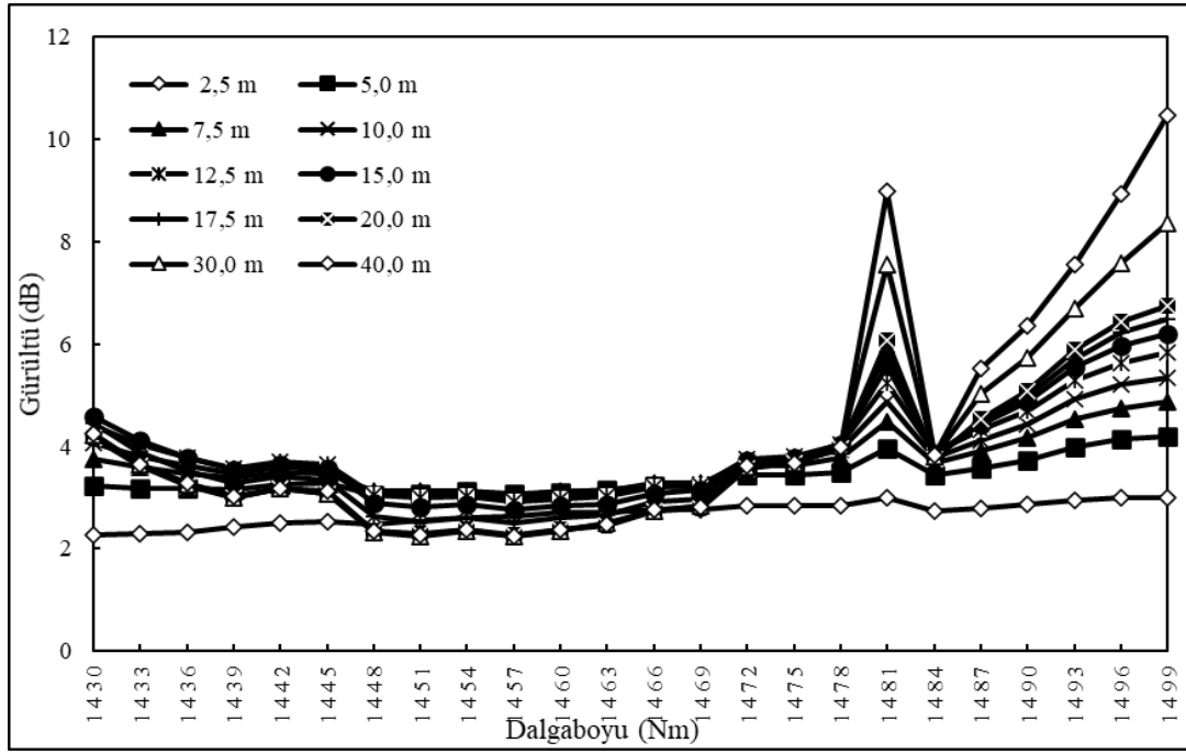
Şekil 5: Farklı TKF uzunluklarında oluşan TKFY gürültü-dalgaboyu grafiği
