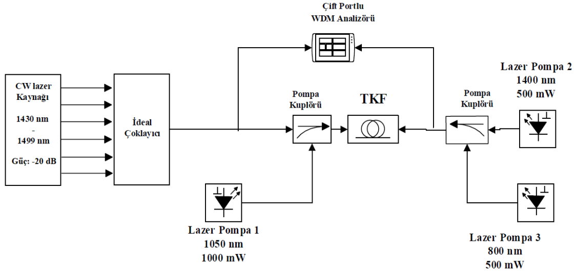
Şekil 3: Çift yönlü üçlü pompalama yapılan TKFY devresi
