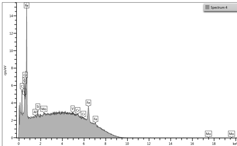
Şekil 2. Geleneksel ısı işlem görmüş numuneye ait EDS analizi
