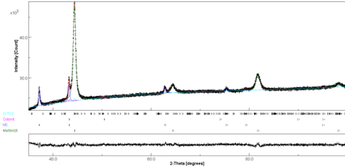
Şekil 4. Geleneksel ısıl işlem görmüş numuneye ait XRD analizi
