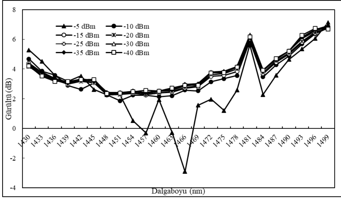
Şekil 9: Farklı giriş güçlerinde oluşan TKFY gürültü - dalgaboyu grafiği
