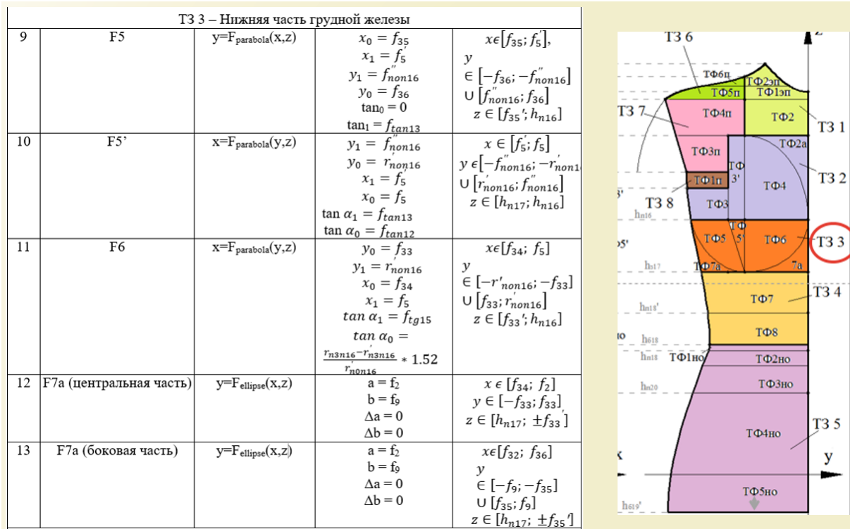
Рис.3 Фрагмент математической модели поверхности фигуры (Fragment of a mathematical model of the shape surface)
