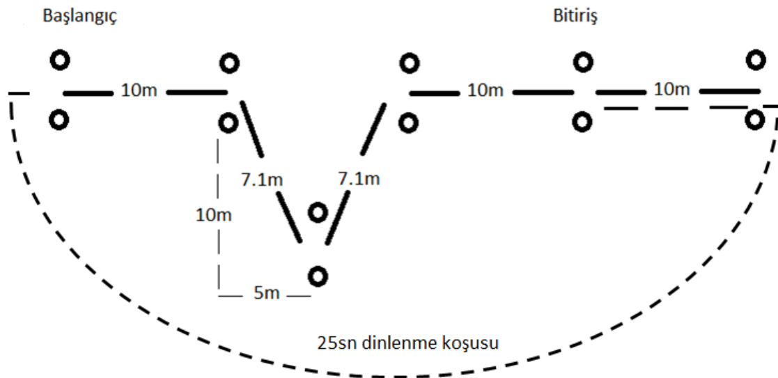
Şekil 2 7 Tekrarlı Yön Değiştirmeli Tekrarlı Sprint Testi
