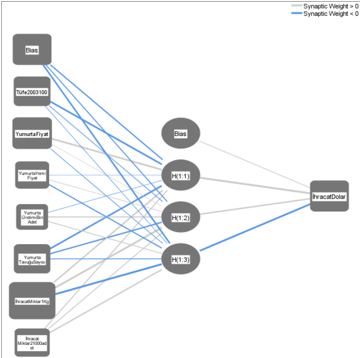
Şekil 4. Tasarlanan MLP Modelinin Mimarisi ve Katmanları
