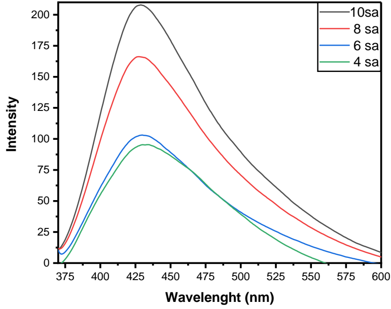
Şekil 1: Sitrik asit ve peçetenin 150 °C’de farklı zaman aralıklarındaki PL (fotolüminesans) spektrumu.
