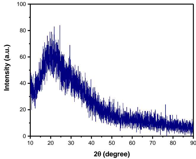
Şekil 4: Sitrik asit ve peçetenin 150 °C’de farklı zaman aralıklarındaki XRD spektrumu.
