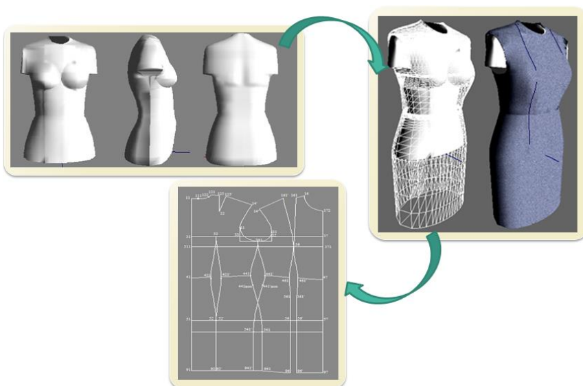
Рис.4 Этапы параметрического проектирования формы и конструкции одежды ( Stages of parametric design of the form and design of clothing )
