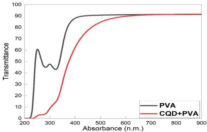
Şekil 6. Saf PVA ve CQD katkılı PVA filmlerin UV geçirgenlik spektrumu
