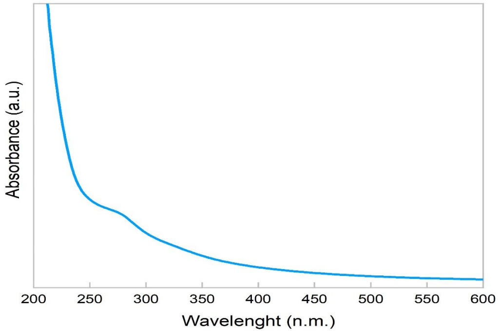
Şekil 1. Balık kılçığından üretilen CQD'lerin UV-Vis absorpsiyon spektrumu
