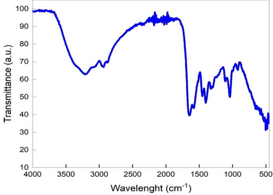
Şekil 3. Sentezlenmiş Karbon kuantum noktaların FT-IR spektrumu
