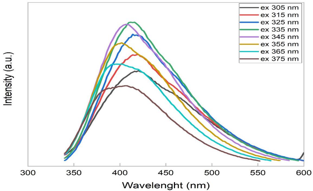
Şekil 2. Sentezlenen Karbon kuantum noktalarının uyarıma bağlı fotoluminesans spektrumları.
