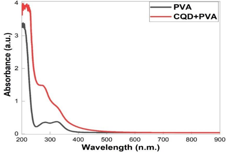
Şekil 5. Saf PVA ve CQD katkılı PVA filmlerin UV absorpsiyon spektrumu
