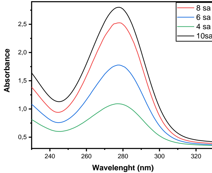
Şekil 2: Sitrik asit ve peçetenin 150 °C’de farklı zaman aralıklarındaki UV spektrumu.
