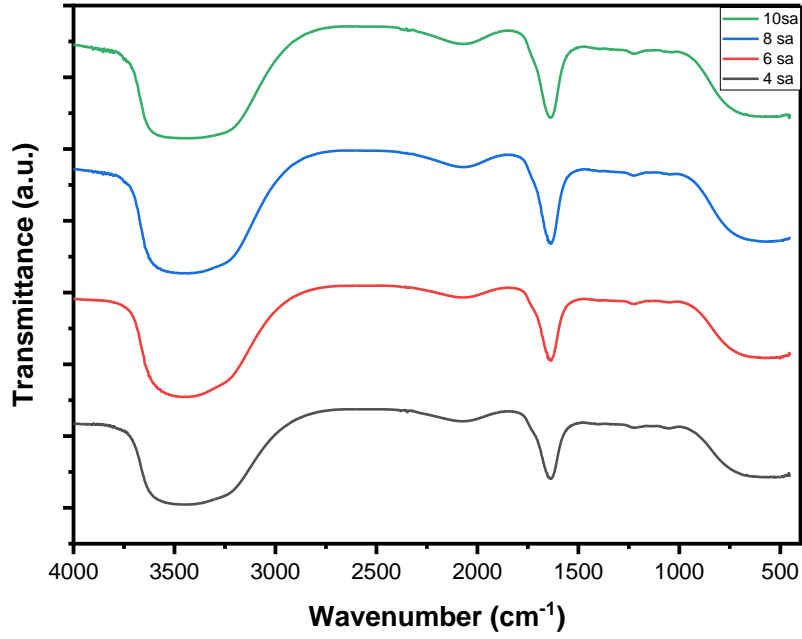
Şekil 3: Sitrik asit ve peçetenin 150 °C’de farklı zaman aralıklarındaki FTIR spektrumu.
